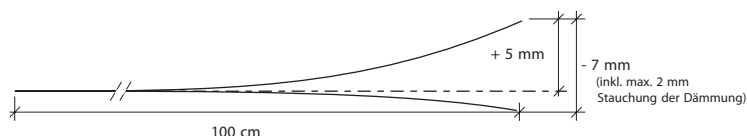
Toleranz Aufwölbungen/Rückbildungen Tolérance déformations/régressions
