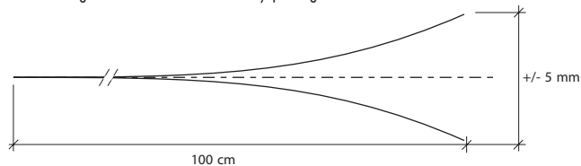
Versatz bei höhengleichen Anschlüssen/Durchgängen
